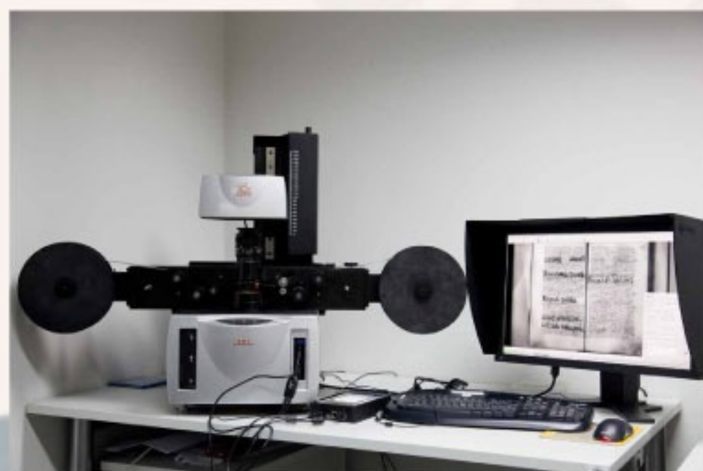
Skaner mikrofilmowy zintegrowany z komputerem, z prawej widoczny monitor, 2009, NAC, 31-196-2
