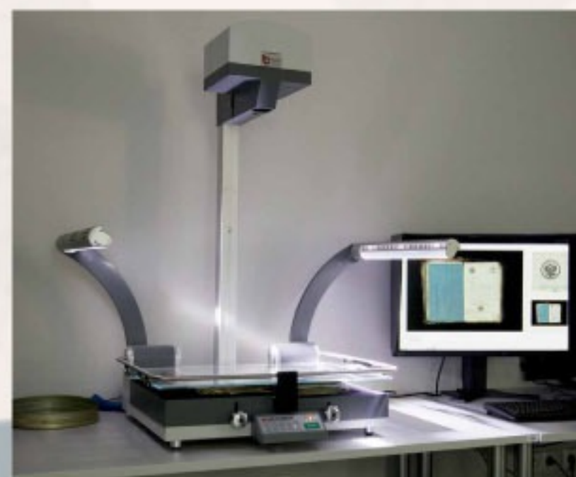
Skaner książkowy do digitalizacji aktowych materiałów archiwalnych, 2009, NAC, 31-196-1
