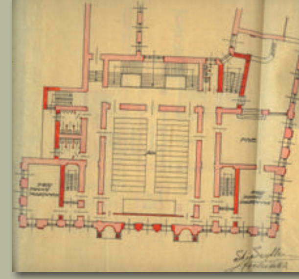
Plan 1. piętra
