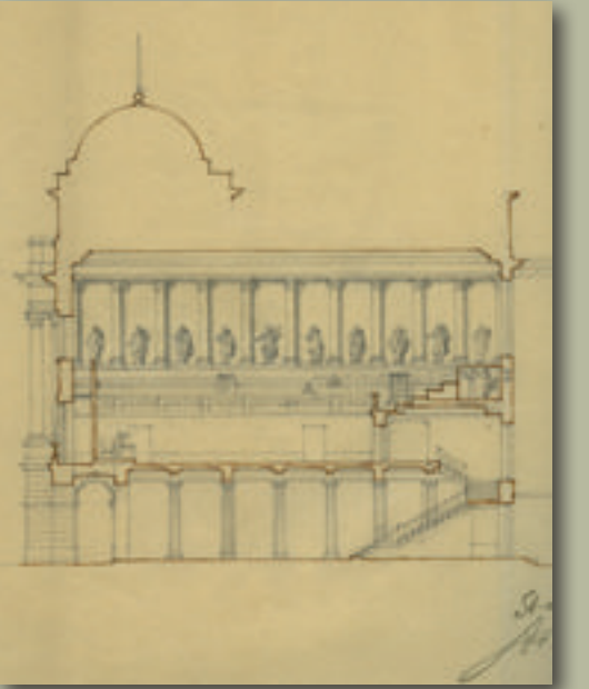
Przekrój
