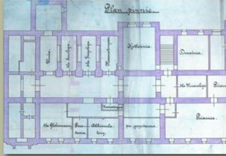
Plan piwnic
