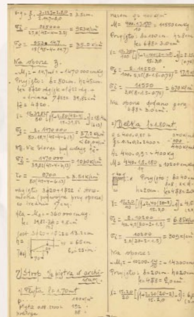
Obliczenia statyczne wytrzymałości stropów żelbetonowych projektowanego gmachu Centralnego Archiwum Państwowego w Warszawie, b.d., AAN, 1919-1990, 64
